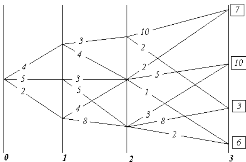
Рис. 4. К существованию метода динамического программирования. Матрица возможностей.
